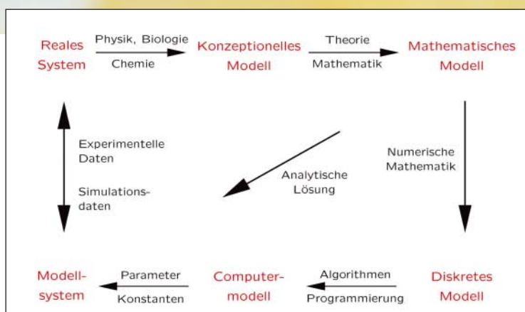
Abb. 1: Formulierung eines Computermodells. Das konzeptionelle Modell wird auf Grund einer konkreten Fragestellung und naturwissenschaftlichen Beschreibung des realen Systems entworfen. Das daraus gewonnene mathematische Modell hat oft nur für Spezialfälle eine analytische Lösung. In allen anderen Fällen muss das Problem numerisch gelöst werden, dazu dienen Computerprogramme. Experimentell gewonnene Erkenntnisse über das reale System werden verwendet um das Computermodell zu optimieren.
