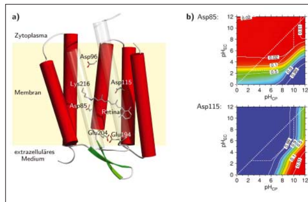
Abb. 3: Bakteriorhodopsin. a) Der Retinalkofaktor ist zwischen den Transmembranhelices des Proteins gebunden. Die geeigneten Aminosäuren sind an der Translokation des Protons über die Membran beteiligt. b) x-Achse: pH im Zytoplasma, y-Achse: pH im extrazellulären Medium. Die Protonierungswahrscheinlichkeiten sind farbkodiert. Asp85 muss deprotoniert sein, damit Protonentransfer vom Zytoplasma ins extrazelluläre Medium stattfinden kann. Bei hohem zytosolischem pH ist aber Asp115 deprotoniert, und Asp85 protoniert.
